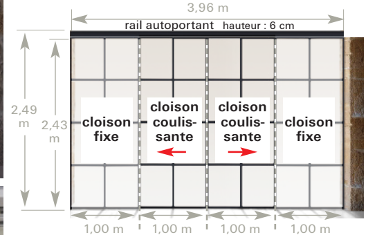
Cloison verrière avec soubassement tôle, carreaux allongés
