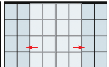
4. Cloison verrière à grands carreaux Cloisons fixes et coulissantes 4 vitres en hauteur. Vitre largeur 46,5 cm, hauteur 57,5 cm
